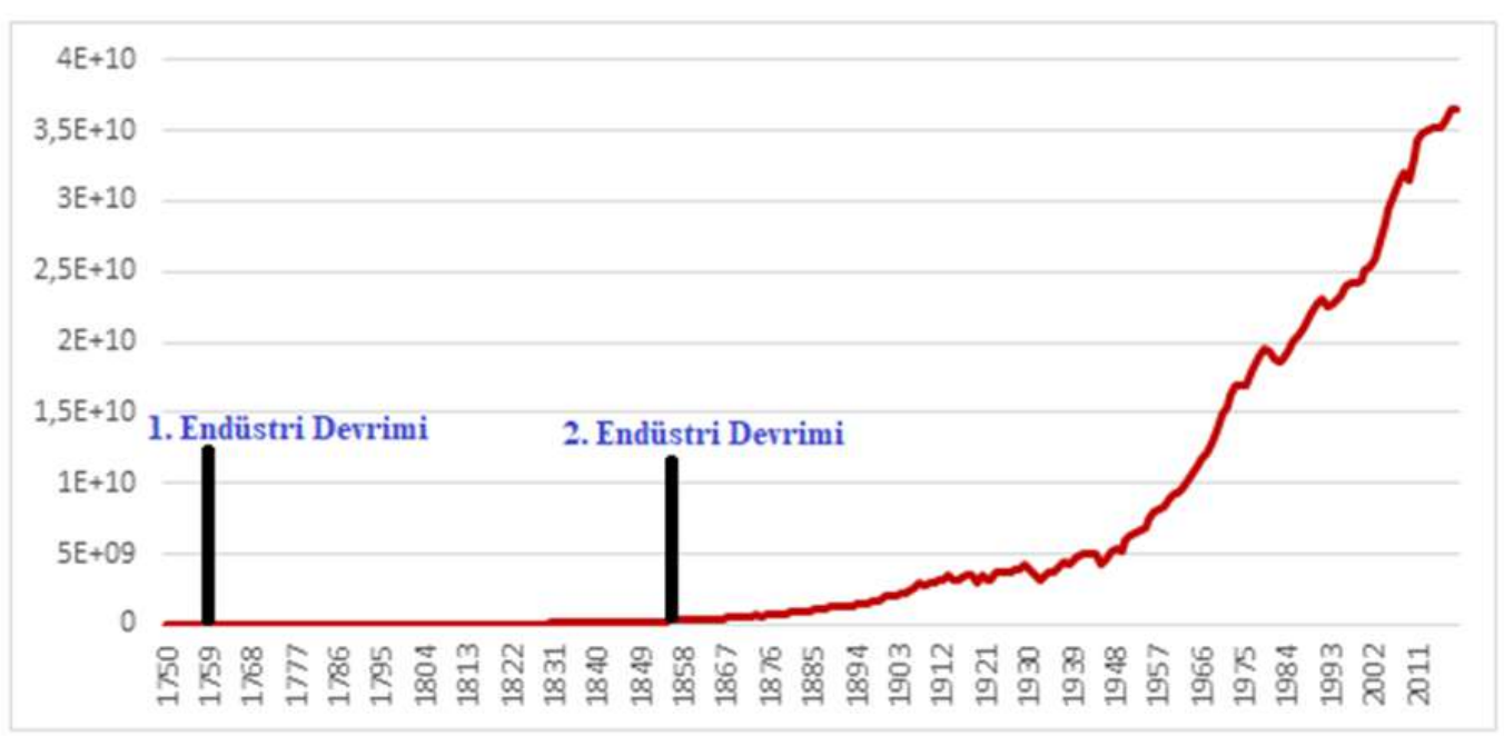
Grafik 1. Tarihsel Olarak Küresel Karbondioksit (CO 2 ) Salım Miktarı
